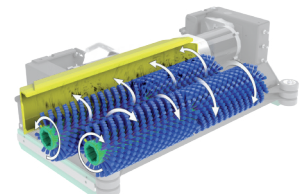
Zylinderbürsten/Brosses cylindriques
