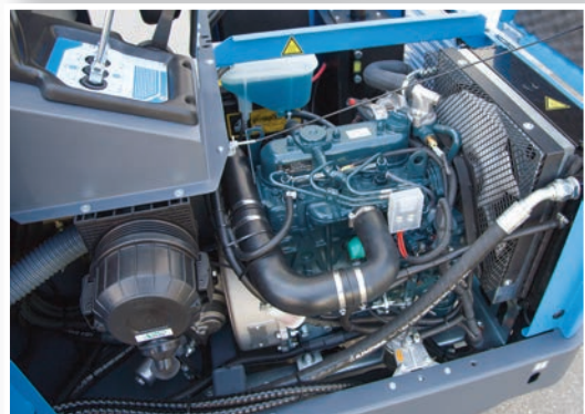
Versione con motore Diesel "Kubota" 4 cilindri raffreddati a liquido Diesel engine "Kubota" version, 4 cyl. liquid cooled
